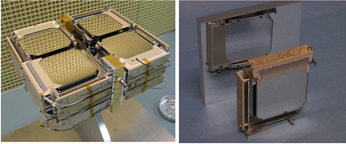
(左) COSI 計畫所研發由 12 片高純度鍺偵測器構成的儀器；(右) 每片偵測器尺寸 8 cm x 8 cm x 1.5 cm，兩面有垂直的條狀電極。
