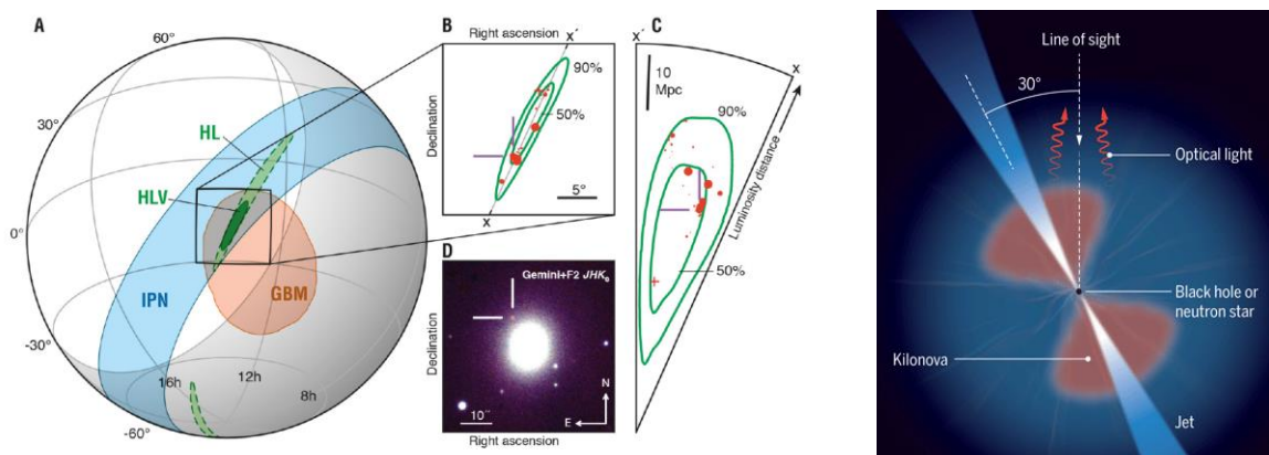
(左) GW170817 重力波源定位，以及最終從 49 個可能星系當中確定所在星系 (Kasliwal et al 2017)；(右) 中子星合併引發重力波與伽瑪線爆發，也產生千級新星而製造大量重元素 (影像取自 Kasliwal et al 2017 「科學」雜誌論文，Science 雜誌網站)。NCU 團隊也參與此次重要發現。
