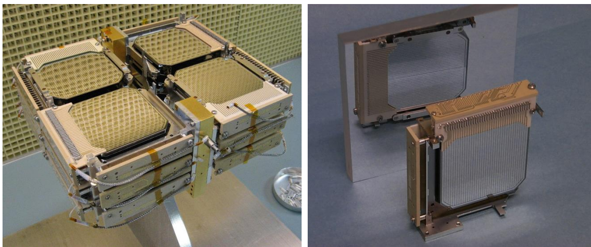
圖 8——（左）COSI 計畫所研發由 12 片高純度鍍偵測器構成的儀器；（右）每片偵測器尺寸 8 cm x 8 cm x 1.5 cm，兩面有垂直的條狀電極。
