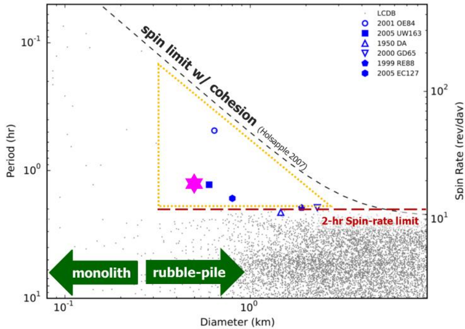
圖3——小行星直徑與自旋週期分布圖。直徑大於數百公尺的小行星有2小時的自旋極限（紅色虛線），否則會因為過大的離心力而崩解。然而有一群「超快自旋小行星」卻能轉得更快（黑色虛線），可能因為內部有黏著力。目前已知六顆超快自旋小行星（藍色符號，其中實心符號為NCU團對所發現）。研究這些超快自旋小行星對能夠幫助我們了解小行星的內部結構（CK Chang）。
