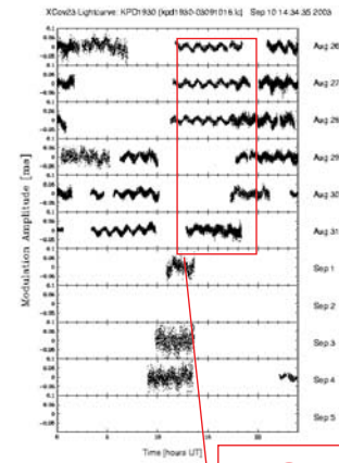
星震觀測
