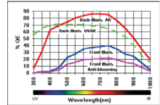
量子效應
